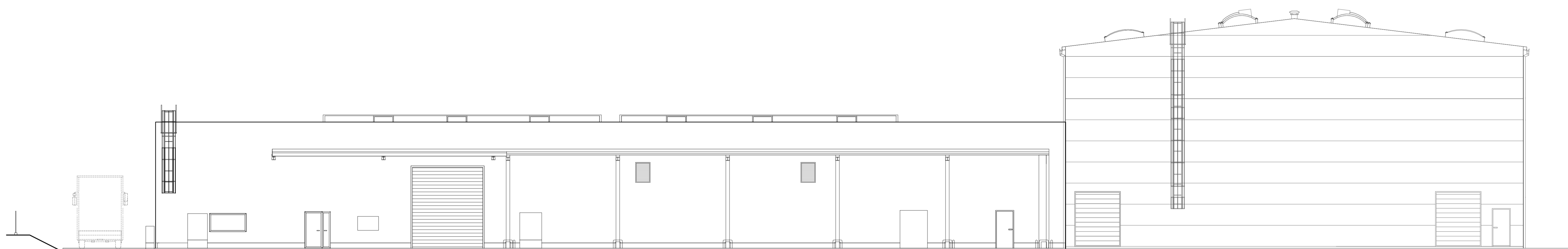
ELEWACJA WSCHODNIA (BOCZNA)
